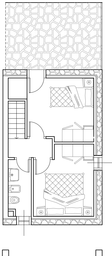
PIANO PRIMO
